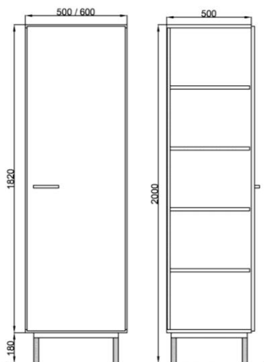
Armoire 1 porte
